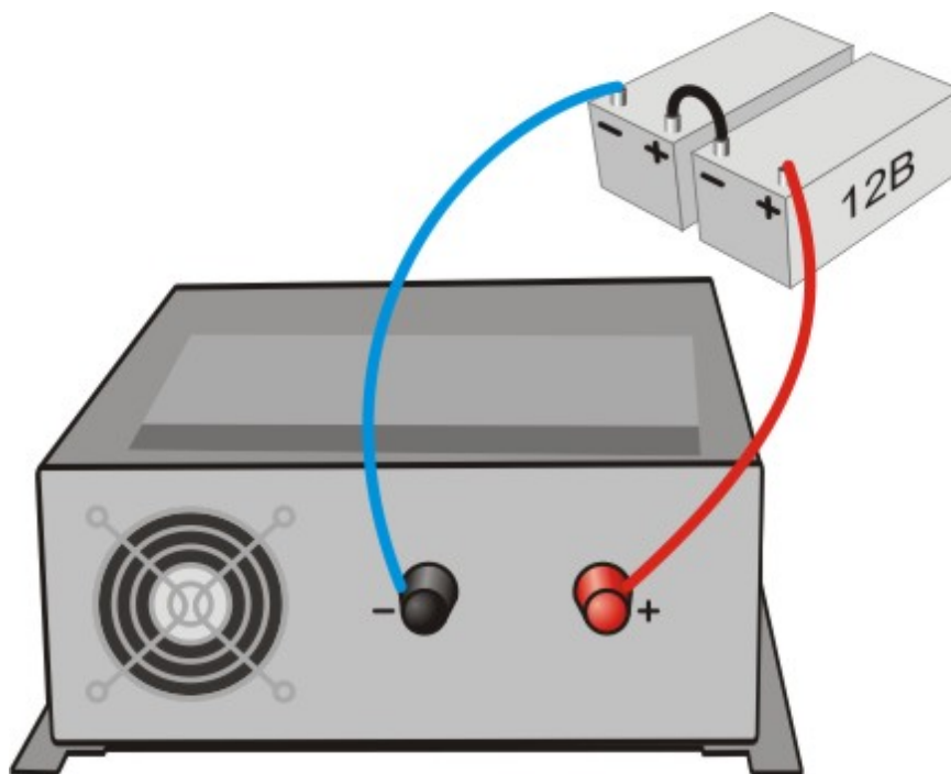
Рис 2. Подключение аккумуляторов к устройству бесперебойного питания
